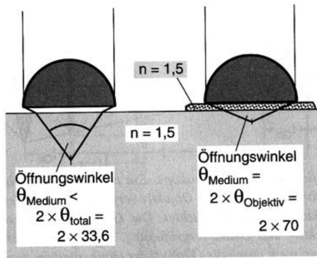
Bild 3.53: Durch den Einsatz einer Immersionsflüssigkeit zwischen Objekt und Mikroskoplinse lässt sich die Lichtstärke und das Auflösungsvermögen des Mikroskops wesentlich verbessern.
