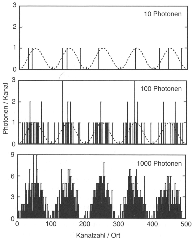
Bild 5.9: Doppelspalt-Experiment im Photonenbild. Oben: werden nur wenige Photonen nachgewiesen, so kann man die Beugungsfigur (gestrichelte Kurve) kaum erkennen. Erst wenn viele Photonen nachgewiesen werden (unten), tritt das Beugungsbild klar hervor.
