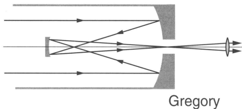
Bild 3.57: Schemazeichnung verschiedener Typen von astronomischen Spiegelteleskopen. Alle Typen wurden im 17. Jahrhundert entwickelt.
