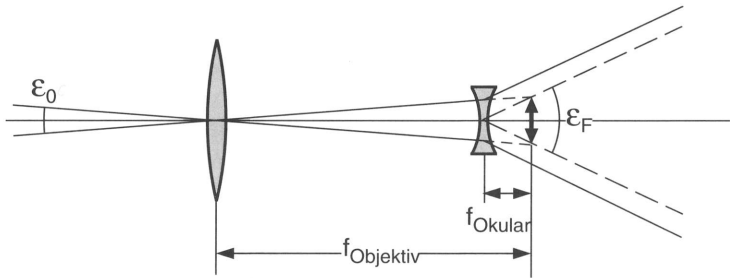
Bild 3.55: Strahlengang in einem terrestrischen Fernrohr.
