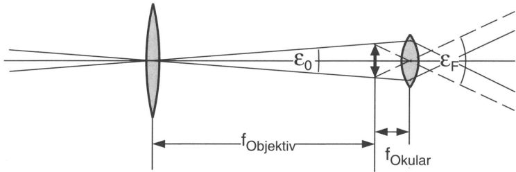
Bild 3.54: Strahlengang in einem astronomischen Fernrohr.
