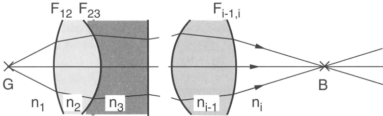
Bild 3.24: Durch mehrfache Anwendung der Abbildungsgleichung lässt sich eine Abbildung durch beliebig komplizierte optische Systeme berechnen.
