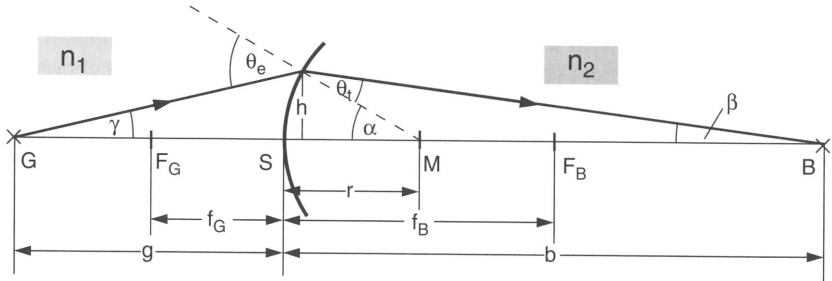
Bild 3.23: Brechung an einer Kugeloberfläche ( M : Mittelpunkt der Kugel), die zwei transparente Bereiche mit Brechungsindex n_1 und n_2 voneinander trennt.
