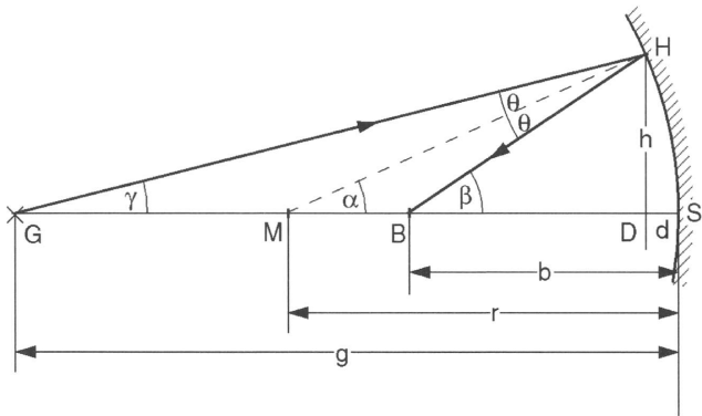
Bild 3.21: Abbildung an einem Kugelspiegel. G : Gegenstandspunkt, M : Kugelmittelpunkt, B : Bildpunkt.
