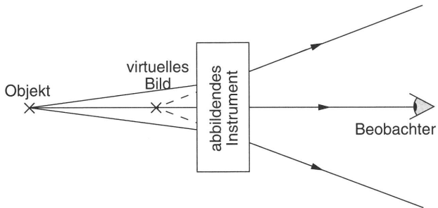
Bild 3.20: Schematische Darstellung einer virtuellen Abbildung. Das abbildende Instrument beeinflusst die Lichtstrahlen so, dass sie dem Beobachter vom Ort des virtuellen Bildes her kommend erscheinen. Ein virtuelles Bild kann nicht mit einem Schirm aufgefangen werden.
