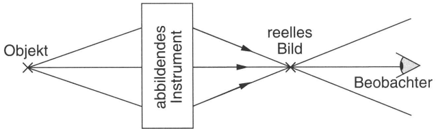
Bild 3.19: Schematische Darstellung einer reellen Abbildung. Das reelle Bild entsteht hinter dem abbildenden Instrument. Es kann direkt beobachtet oder von einem Schirm aufgefangen werden.
