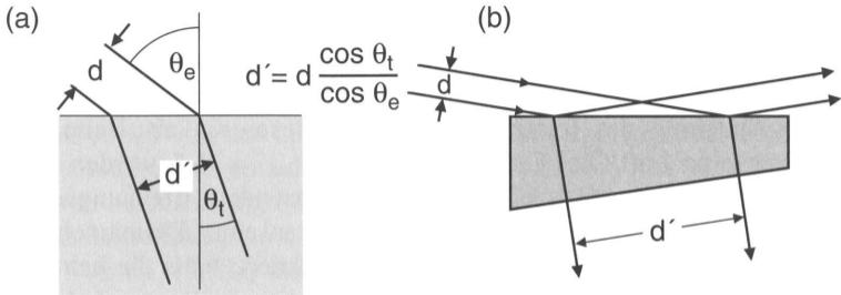
Bild 2.14: Änderung des Bündelquerschnitts bei Brechung (a) und die Möglichkeit, diesen Effekt zur Aufweitung des Bündelquerschnitts zu verwenden (b).
