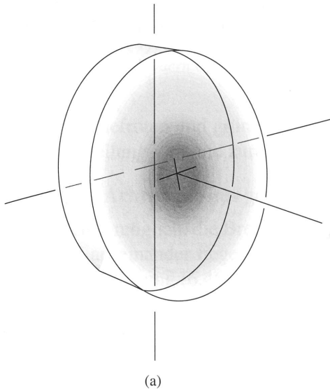
Bild 6.42: Eine Glasscheibe, deren Brechungsindex radial vom Mittelpunkt aus abnimmt. (b) Fokussierung paralleler Strahlen durch eine GRIN-Linse.
