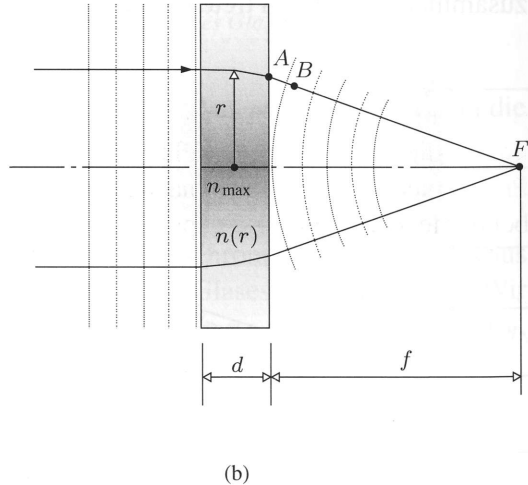
Bild 6.42: Eine Glasscheibe, deren Brechungsindex radial vom Mittelpunkt aus abnimmt. (b) Fokussierung paralleler Strahlen durch eine GRIN-Linse.
