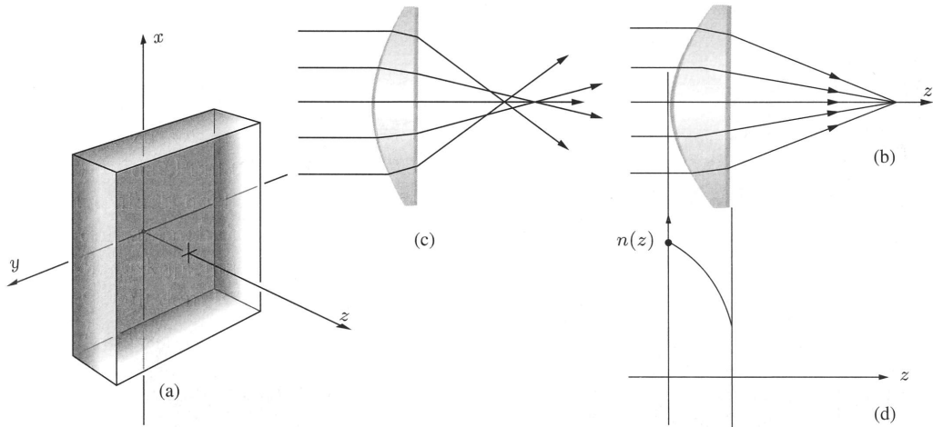
Bild 6.45: (a) Eine Scheibe axialen GRIN-Materials mit dem Brechungsindex n(z) . (b) Eine axiale GRIN-Linse ohne sphärische Aberration. (c) Eine herkömmliche Linse mit sphärischer Aberration. (d) Das Profil des Brechungsindex.
