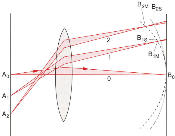
Abb. 9.46. Bildfeldwölbung
