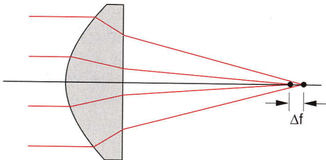
Abb. 9.40. Unterschiedliche sphärische Aberration bei den zwei verschiedenen Orientierungen einer plan-konvexen Linse
