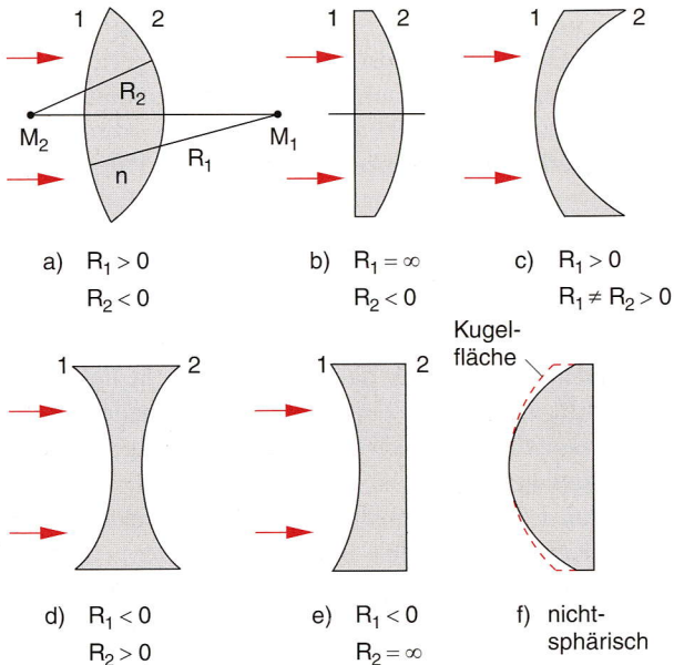
Abb. 9.25a-f. Beispiele für verschiedene Linsenformen. (a) konvex-konvex = bikonvex, (b) plan-konvex, (c) konvex-konkav, (d) bikonkav, (e) konkav-plan, (f) nichtsphärische Linse
