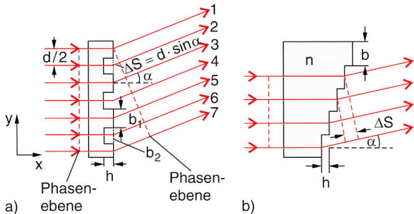
Abb. 12.31. (a) Beugung von Licht an einem streifenförmigen Phasengitter, (b) Ablenkung von Licht durch eine Stufenplatte
