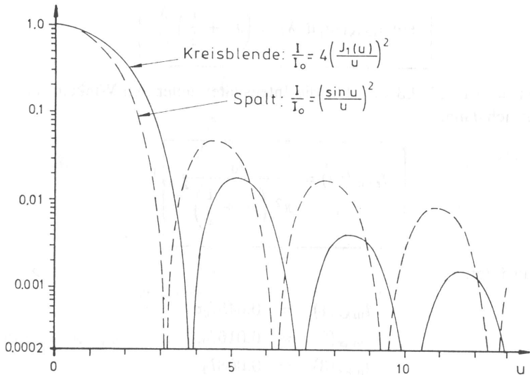
Bild 1.7 Beugung bei Spalt und Kreisblende
