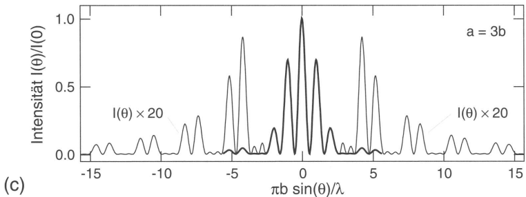
Bild 4.19: Doppelspalt – (a) und (b) schematische Darstellung; (c) Intensitätsverlauf für einen Spaltabstand a = 3b .
