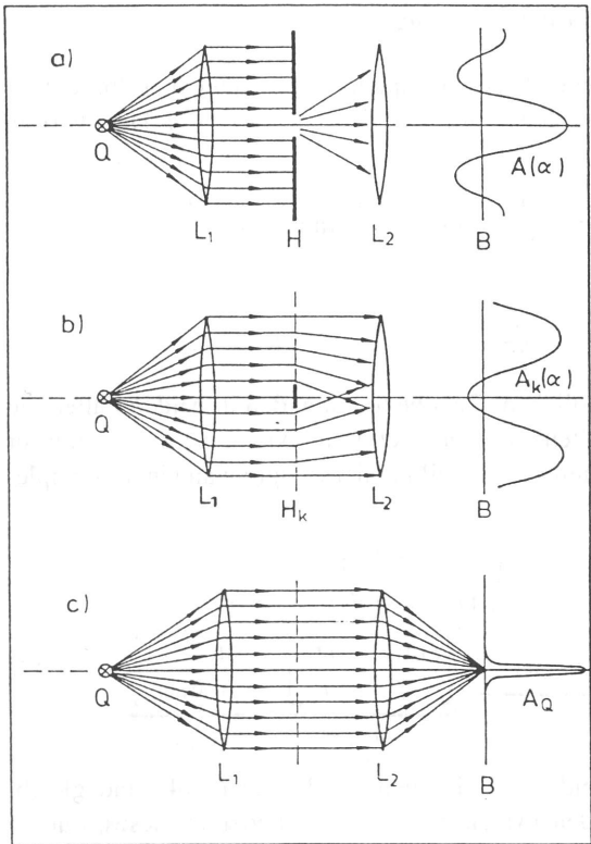
Bild 1.16 Zum Babinetschen Theorem
